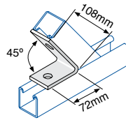
45° Acute Angle 'T' Bracket
