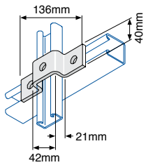
Top Hat
