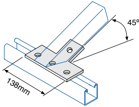
45° Acute Angle 'T' Bracket
