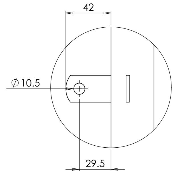
LUGS SCALE 1 : 2
